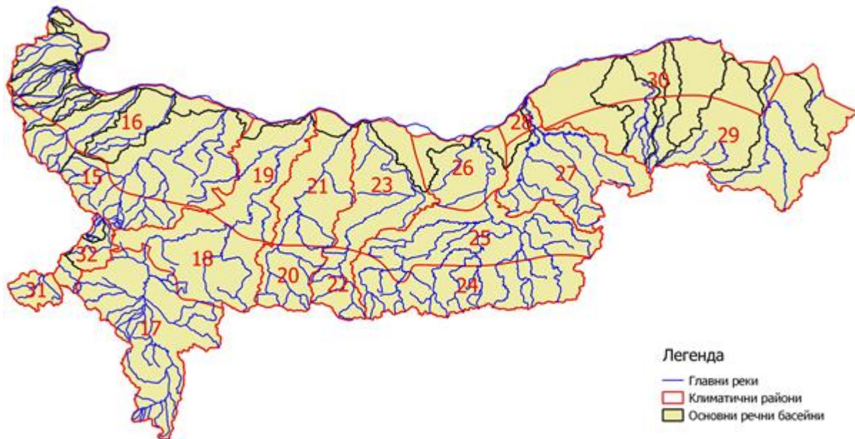
Фигура 3. Основни речни басейни и Райони за оценката на натиска и въздействието върху повърхностните и подземните води от изменението на климата в Дунавски район
