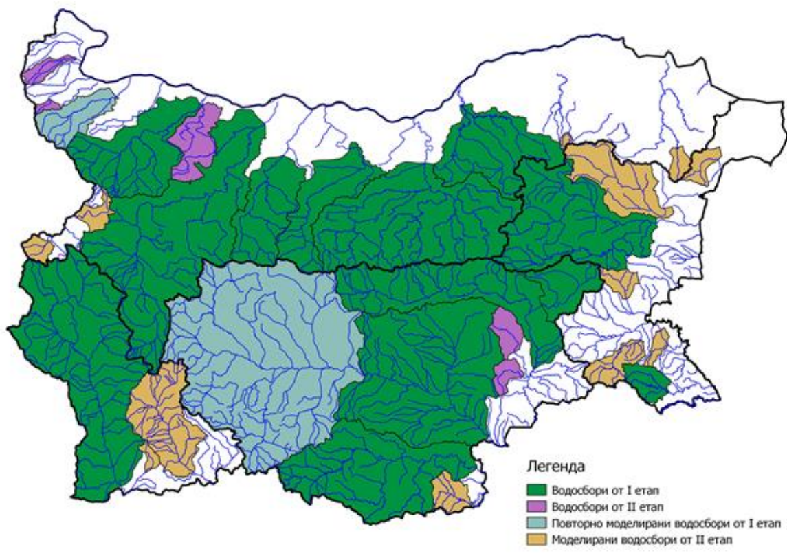
Фигура 1. Моделирани водосбори
