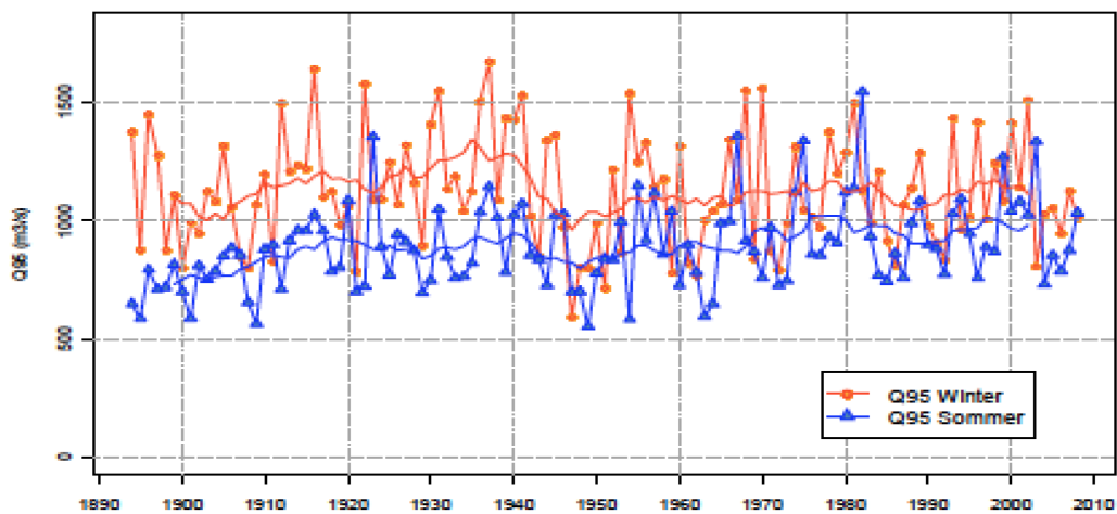
Abbildung 5-12: Zeitreihe der saisonalen Niederwasserdurchflüsse (Winter Q_{95} u. Sommer Q_{95} ) am Pegel Donauebenfurt für die Periode 1893-2008.
