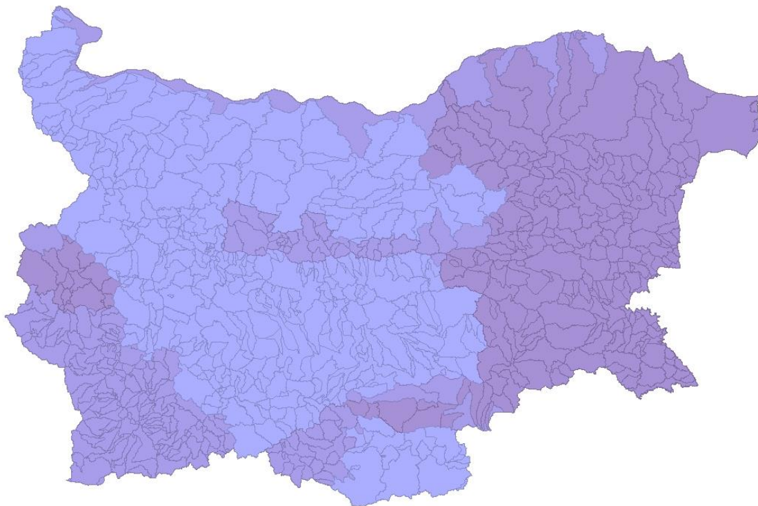
Фигура 2.2.5.3. Интензивност на очакваните климатични промени за периода 2071-2100 г. за сценарий RCP 8.5.
