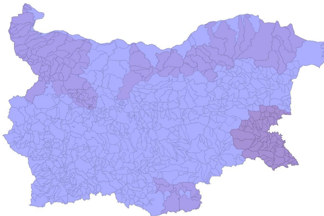
Фигура 2.2.5.1. Интензивност на очакваните климатични промени за периода 2013-2042 г. за сценарий RCP 8.5.
